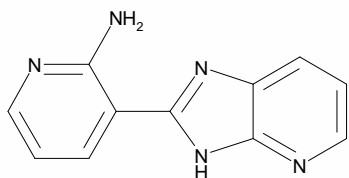
2-(2-Amino-3-pyridyl)-7-azabenzimidazole
