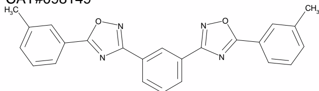
1,3-Bis[3-(3-tolyl)-1,2,4-oxadiazolyl]benzene
