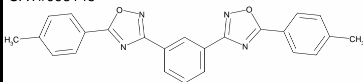
1,3-Bis[3-(4-tolyl)-1,2,4-oxadiazolyl]benzene
